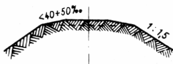
Linie jednotorowe w nasypie
