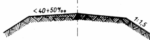
Linie dwutorowe w nasypie
